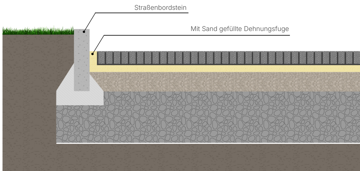
Abbildung 3 Dehnungsfuge am Bordstein
