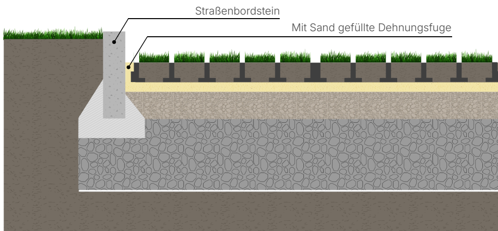
Abbildung 3 Dehnungsfuge am Bordstein
