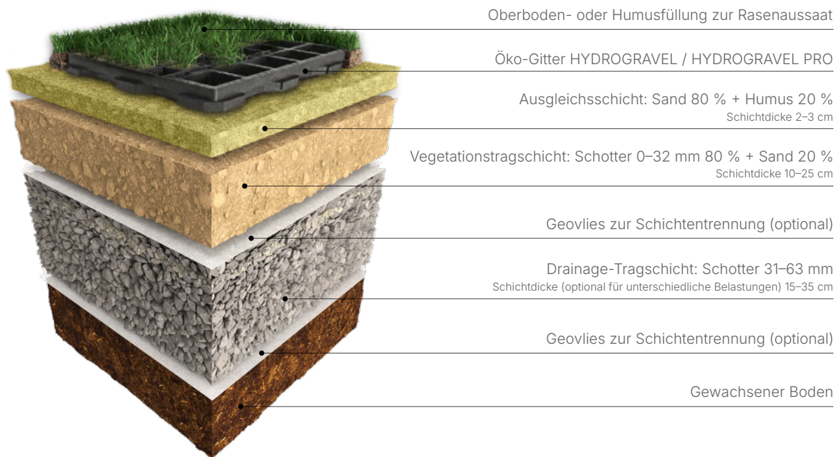
Abbildung 5 Empfohlene Schichten des Unterbaus
